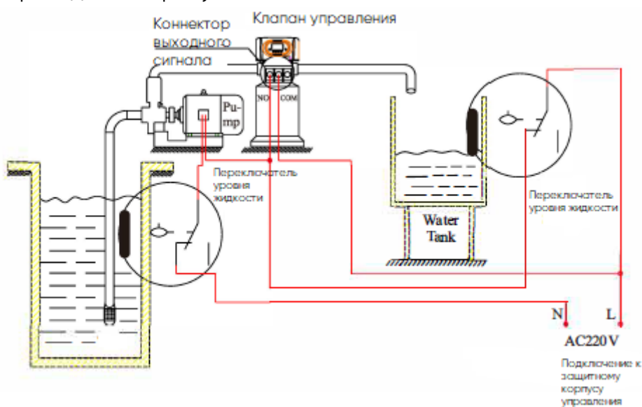
Рисунок 3-5 Подключение контроллера уровня жидкости, управляющего впускным насосом
