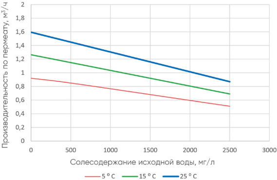
Расчетный график зависимости производительности одной мембраны от общего солевого содержания при заданных температурах*
