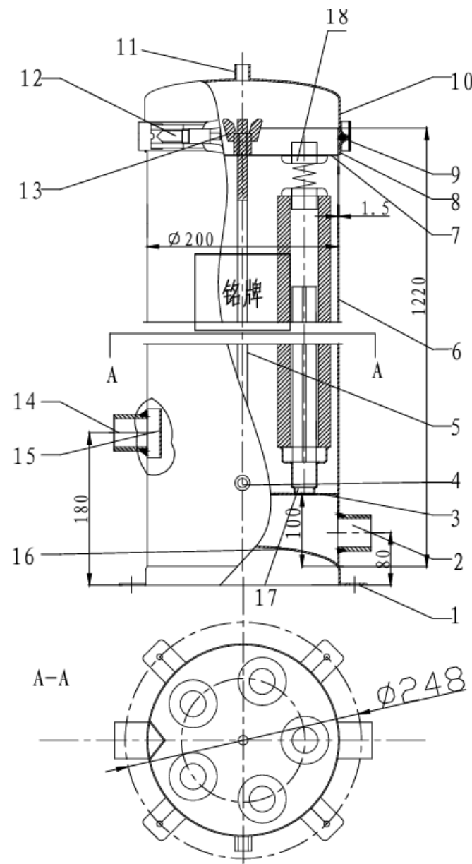
Спецификация оборудования: Мультипатронный фильтр тонкой очистки воды, модель АК CF 5x40
