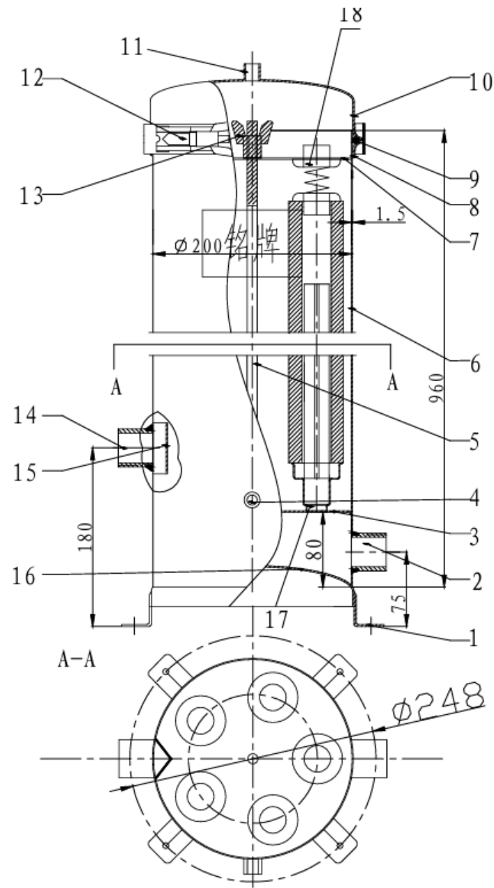
Спецификация оборудования: Мультипатронный фильтр тонкой очистки воды, модель АК CF 5x30
