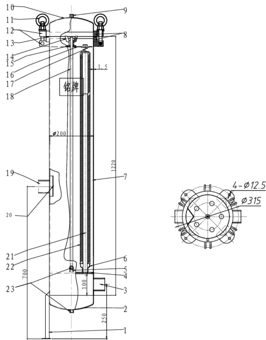
Спецификация оборудования: Мультипатронный фильтр тонкой очистки воды, модель АК CF 5x40 (Фланцевое соединение)
