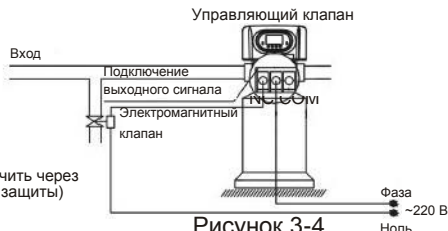
Рисунок 3-4. Подключение через порт сброса давления
