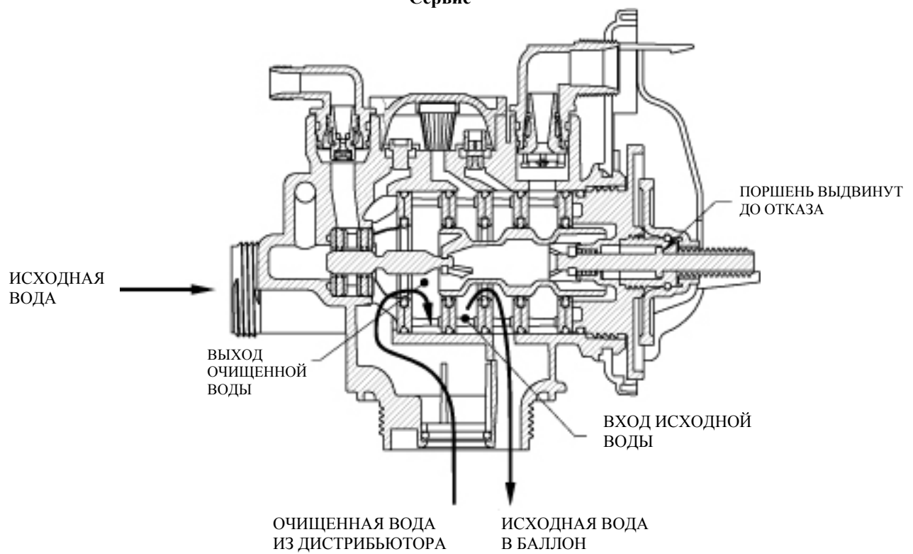
Рисунок 1 Диаграмма потоков в режиме... Сервис
